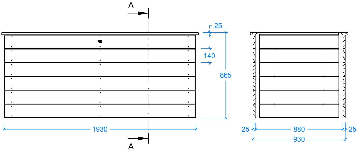
A-A (1:20)
